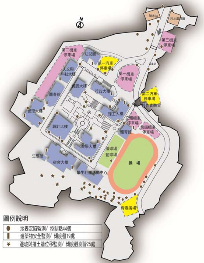
校園建築暨地文監測點分布圖
