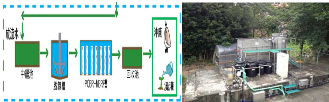
中水回收設施處理流程及設施實景
