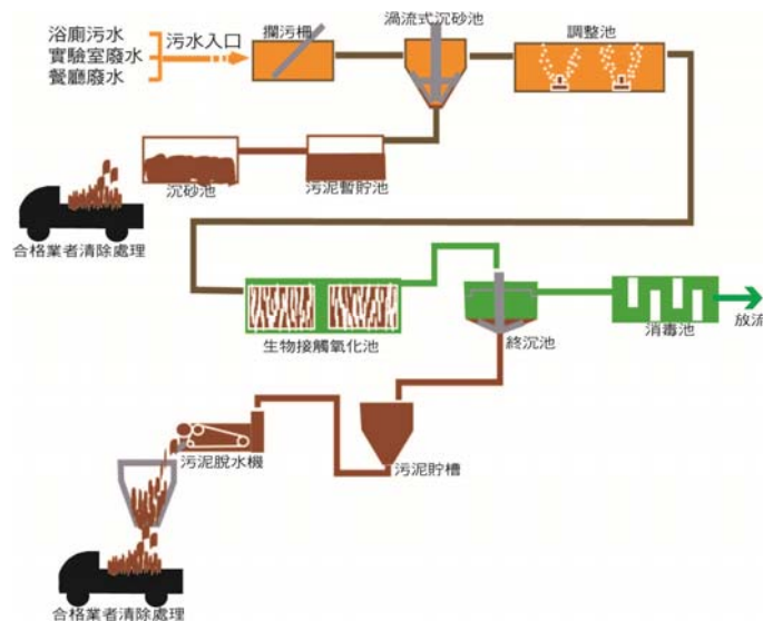
廢水處理流程
