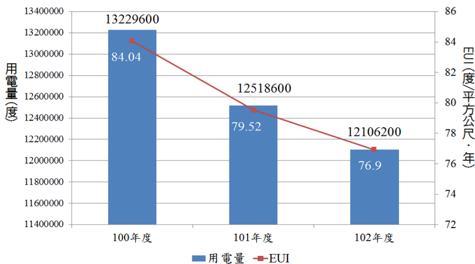
100-102 年校區總用電量與 EUI 比較
